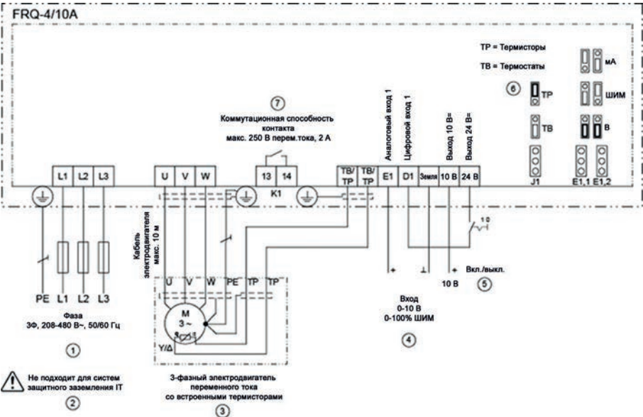
Схема электрических подключений FRQ5 4/10/16A
