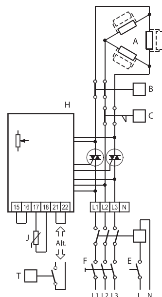
CBM-3 400В 3~
