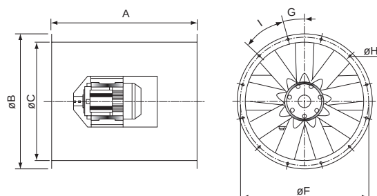
AXCBF 630 - AXCBF 800
