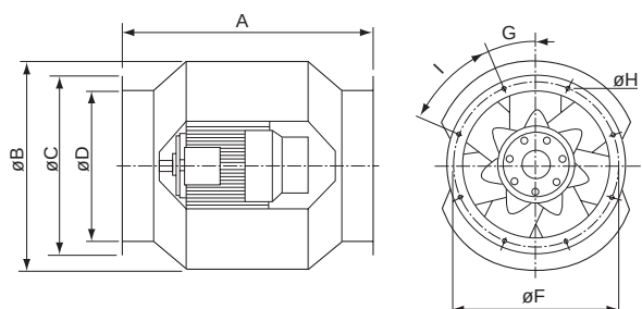
AXCBF 250 - AXCBF 500
